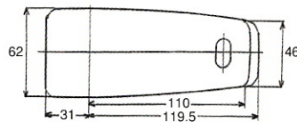
DEL-10A 寸法図
